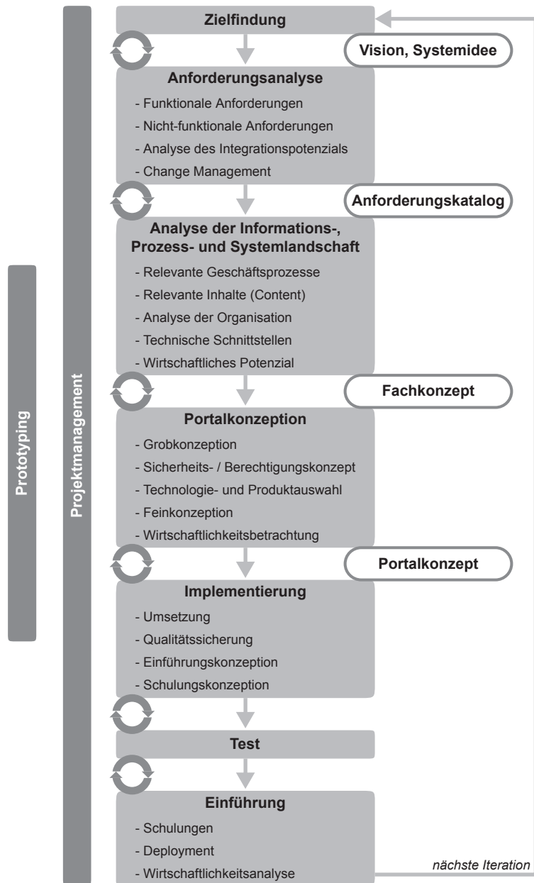
Abbildung 12.2: Vorgehensmodell für Portalprojekte
